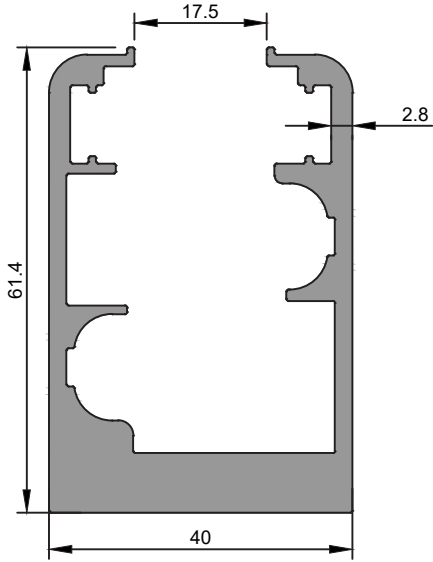
2574 Küpeşte Profil 1,490 kg/m
