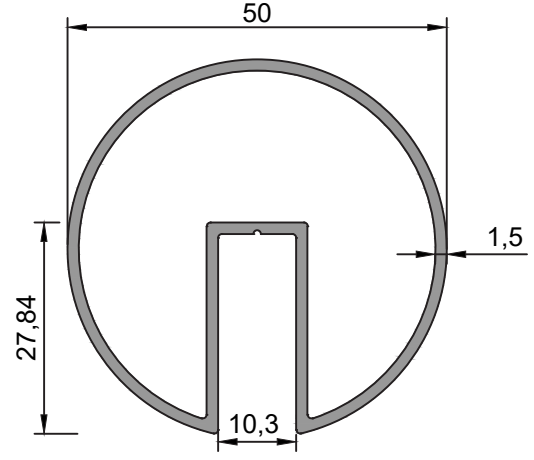
2054 Küpeşte Profili 0,832 kg/m
